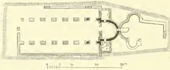
Fig. 4. Doppelbasilika der Symphorosa. (Nach Stevenson.)
