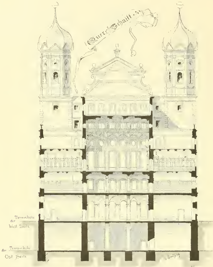
Fig. 4. Querschnitt.
