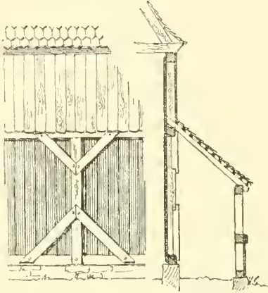
Fig. 3. Konstruktion der Holzkirche zu Braumau.
