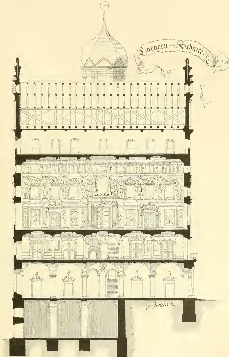
Fig. 3. Längenschnitt.
