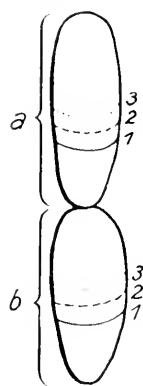
Schema 3.
