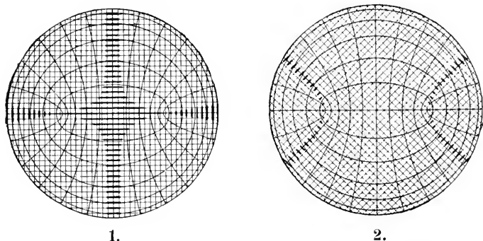
1. Dunkle Balken in Normalstellung. 2. Dunkle Balken in Diagonalstellung. Nach TSCHERMAKs Lehrbuch d. Mineral., 6. Aufl., p. 223.
