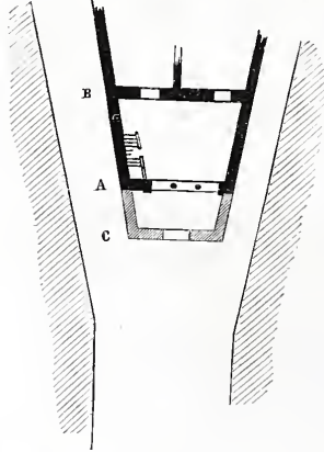
Situationsplan des Albergo del Driso.
