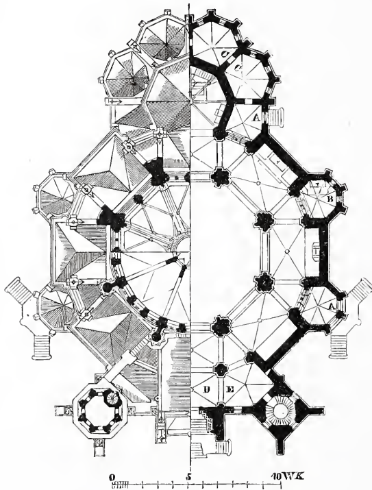
Grundriß der neuen Kirche zu Fünfhaus.
