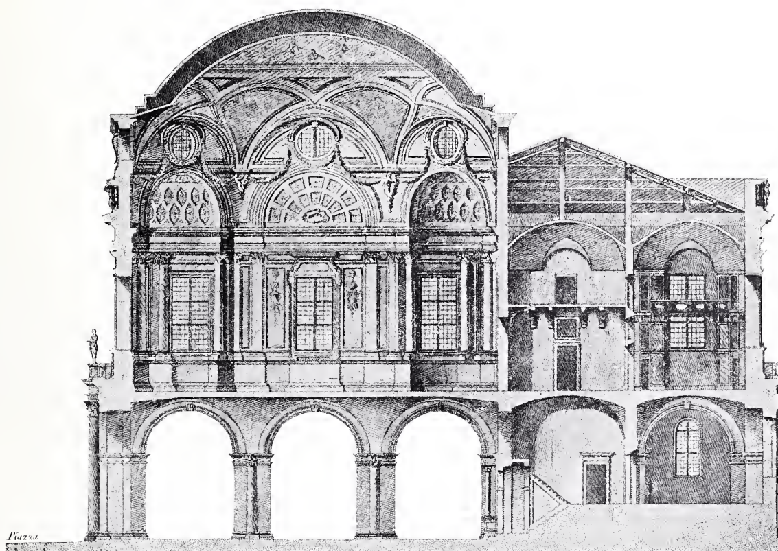
Spaccato per il lungo di tutta la Fabbrica, e Prospetto interiore della gran Sala Moderna
