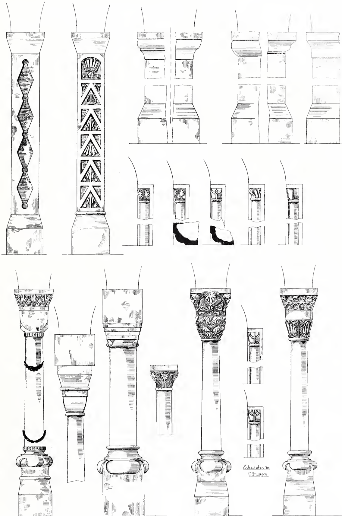
ABB. 11. EINZELHEITEN DER ARCHITEKTUR AUS DER KRYPTA UND DEM KREUZGANG DER MORITZBERGER KIRCHE
