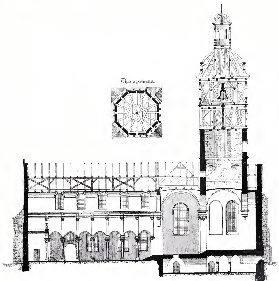
ABB. 3. SCHNITT DURCH DIE MORITZBERGER KIRCHE
