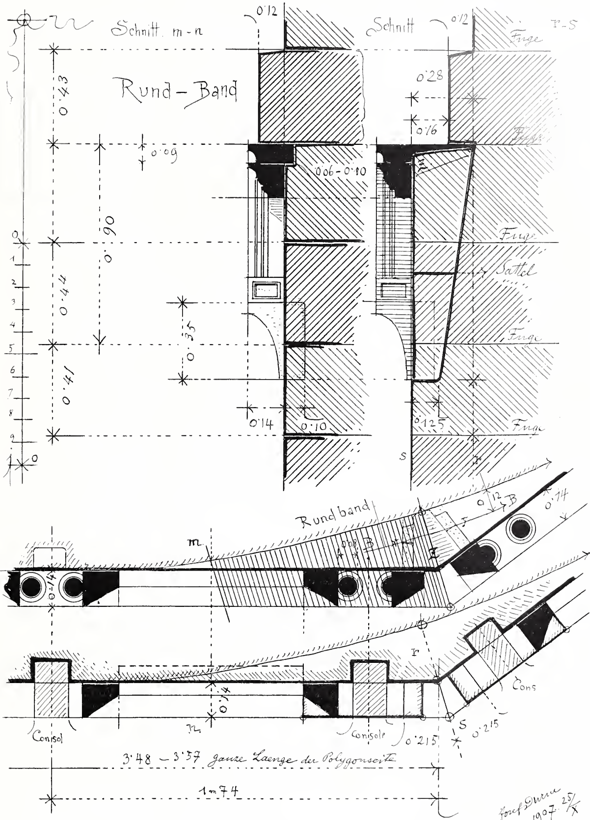
Grabmal des Theoderich. Konstruktion, wie sie sich nach der von Professor A. Haupt vorgeschlagenen Verbrämung mit einem ornamentierten Bogenfries auf Konsolen ergeben würde.
