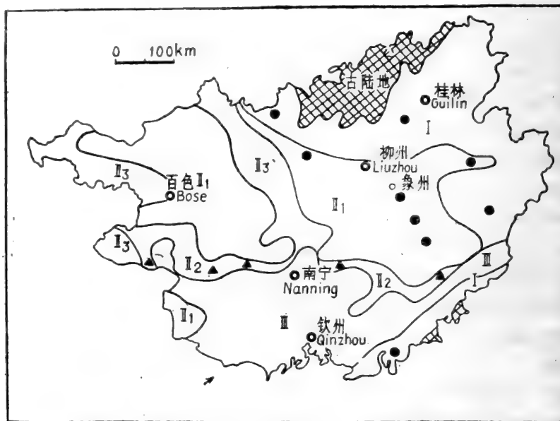
插图 3 广西早泥盆世晚期腕足动物群分布图
