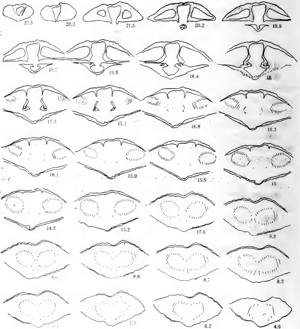
插图 8 Otospirifer shipaiensis Hou et Xian 连续横切面图 (Transverse serial sections of Otospirifer shipaiensis Hou et Xian), ×1.2
