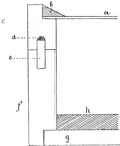
Рис. 208. Схема устройства сложныхъ пазовъ ящичка. a — стекло, b — замазка, c — деревянная стѣнка крышки, d — ватная прокладка, e — деревянный или картонный пазъ, f — деревянная стѣнка ящичка, g — дно, h — торфяная или пробковая настилка ящичка. \frac{1}{1} . По NIERELT'у.
