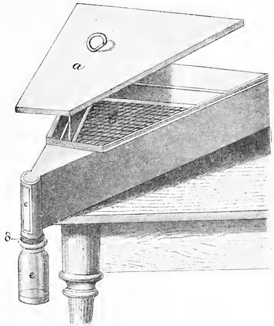
Рис. 191. Фотэциклоторъ. \frac{1}{10} . По Ортнеру. а — крышка, б — стѣкла-перегородка, с — оконце, d — пробочное кольцо, е — банка.
