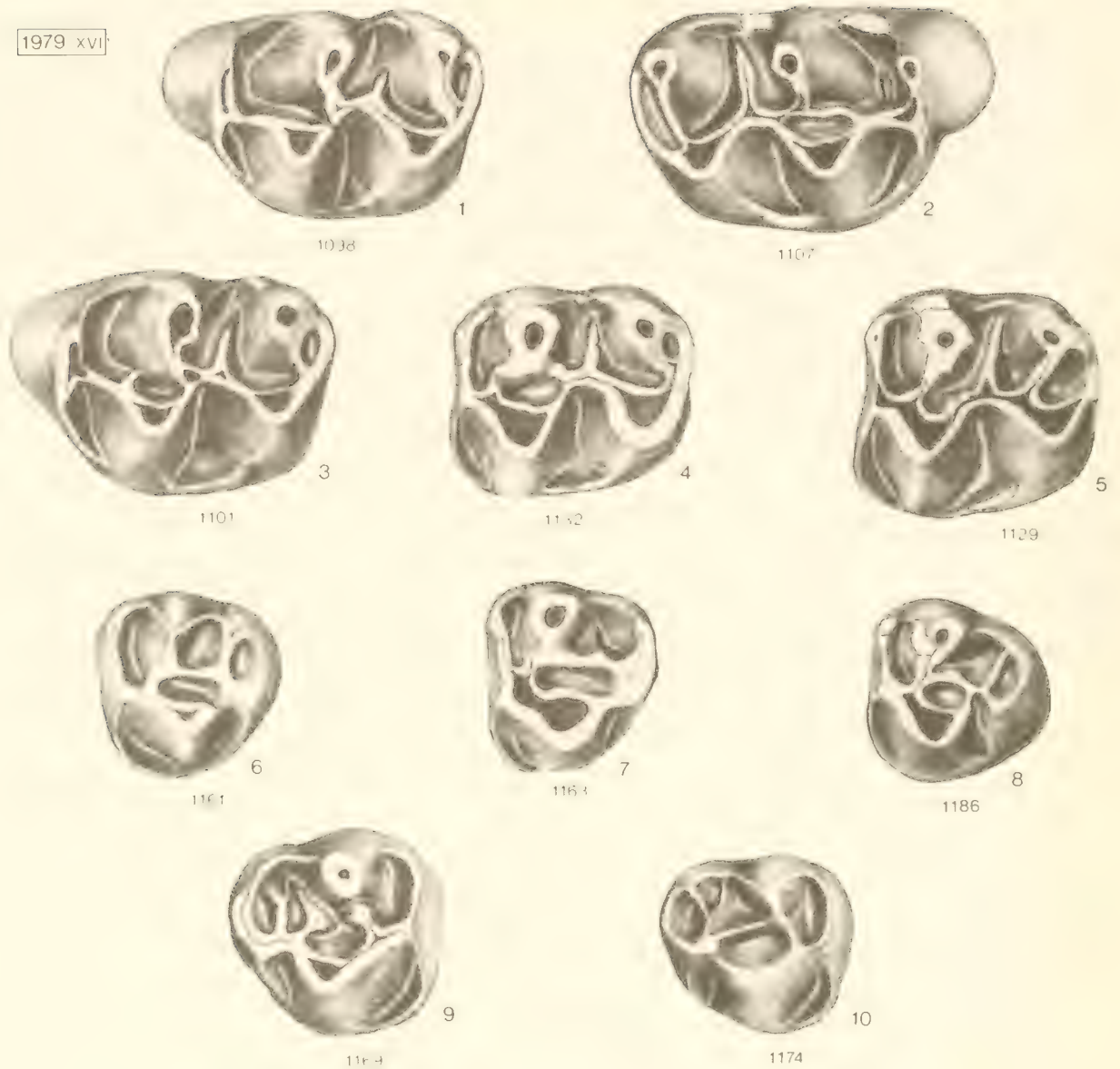
Abb. 5: Democricetodon mutilus FAHLBUSCH aus Puttenhausen. Obere Molaren: li. M 1 (1, 3), re. M 1 (2); li. M 2 (4-5); li. M 3 (6-8), re. M 3 (9-10). ×25
