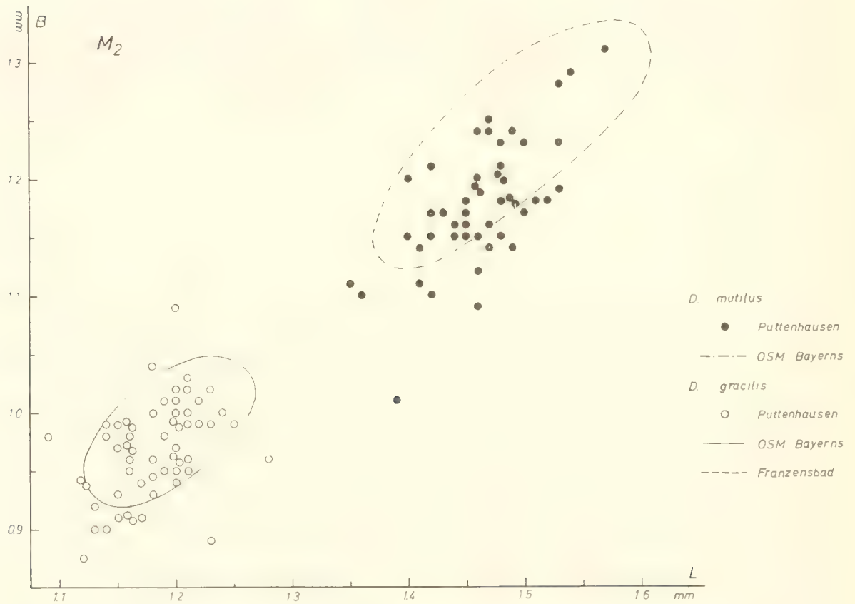
Abb. 3: Längen-Breiten-Diagramme von Democricetodon gracilis FAHLBUSCH und Democricetodon mutilus FAHLBUSCH aus Puttenhausen. Zum Vergleich die Variationsbereiche der beiden Arten aus der OSM Bayerns (nach FAHLBUSCH 1964) und Franzensbad (nach FEJFAR 1974).
