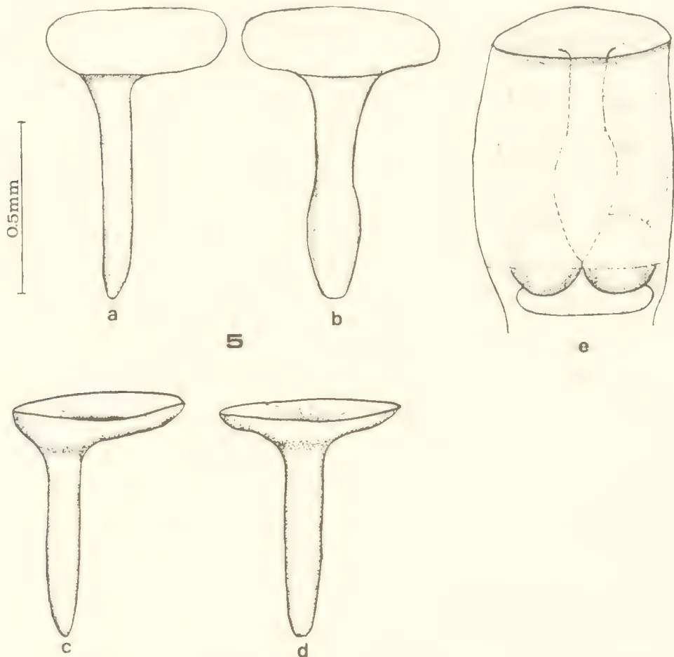
Abb. 5. Janua (Dexiospira) quasiacuta n. sp. a, b. Operculum mit dicker, leicht konvexer Deckelplatte und im proximalen Teil leicht verbreiterten Stiel, c, d. Holotypus (BSP 1978 XX 7) mit konkav eingesenkter Deckelplatte, e. Brutapparat von J. (D.) preacuta VINE nach KNIGHT-JONES, KNIGHT-JONES & KAWAHARA (1975, Fig. 4 E), etwa konvergent dürfte der Brutapparat von J. (D.) quasiacuta n. sp. ausgesehen haben.
