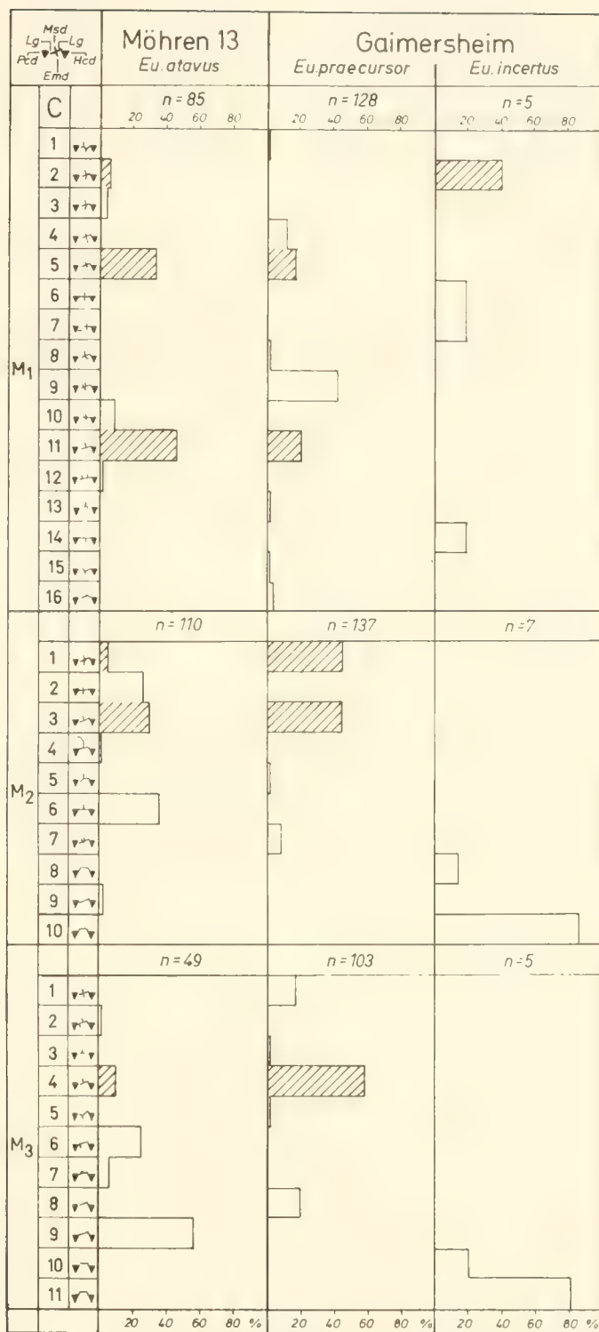
Abb. 12: Strukturelemente der mittleren Quartäler der Unterkiefermolaren von Eurcietodon atavus (Möhren 13), E. praecursor (Gaimersheim) und E. incertus (Gaimersheim). Vergleich der Häufigkeitsverteilungen.
