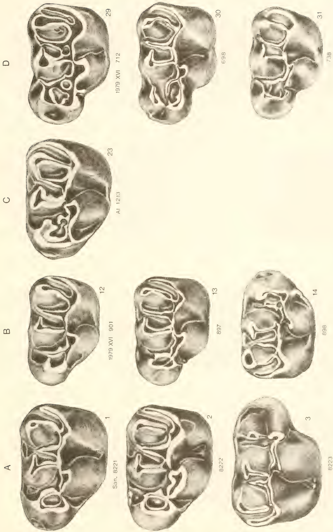
Abb. 14: Die Molaren von Eumyarion medius aus Sansan (A 1-11), E. cf. weinfurteri aus Putttenham (12-22), E. cf. latior aus Anwil (C 23-28) und E. bifidus aus Putttenham (D 29-39). \times 25 Mit Ausnahme von A 3 (re. M 1 ), A 7 (re. M 3 ) und B 14 (re. M 1 ) sind alle Zähne linke.
