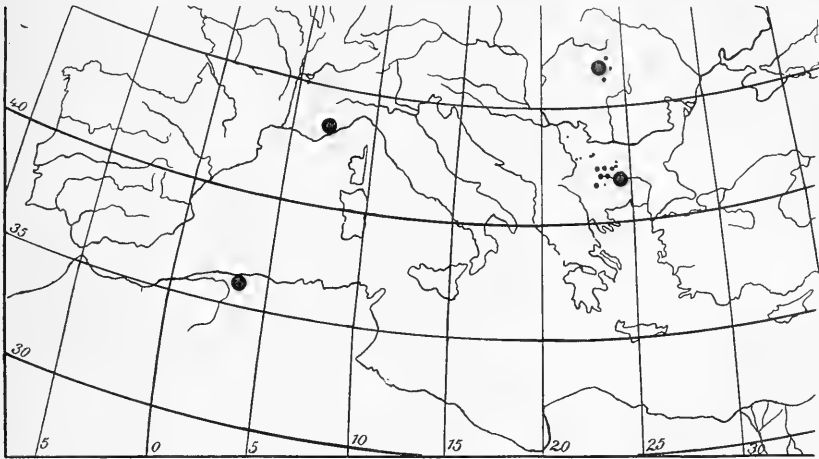
Fig. F. Verbreitungsgebiet des Diptomus lilljeborgi .
