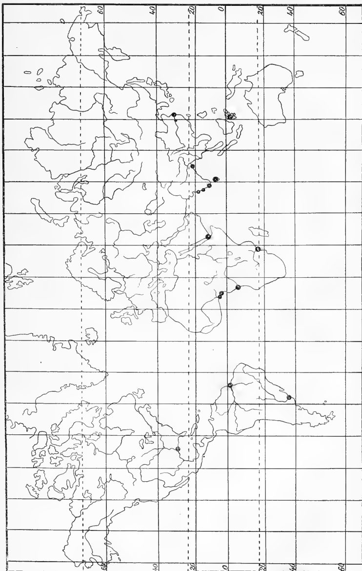
Fig. P a . Verbreitungsgebiet des Genus Pseudodiaptomus .
