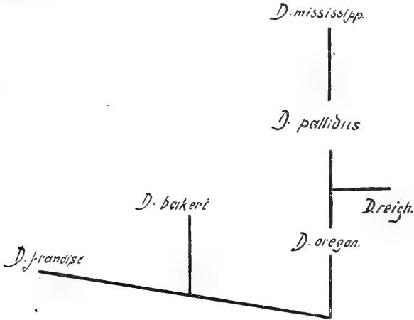
Fig. H 1 . Verwandtschafts-Diagramm der oregonensis -Gruppe.
