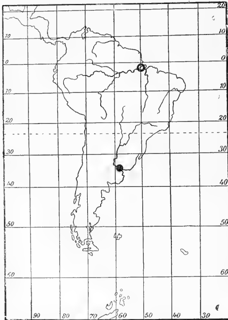
Fig. N o . Verbreitungsgebiet von Pseudodiaptomus gracilis , Diaptomus michaelseni und Pseudoboeckella longicauda .
