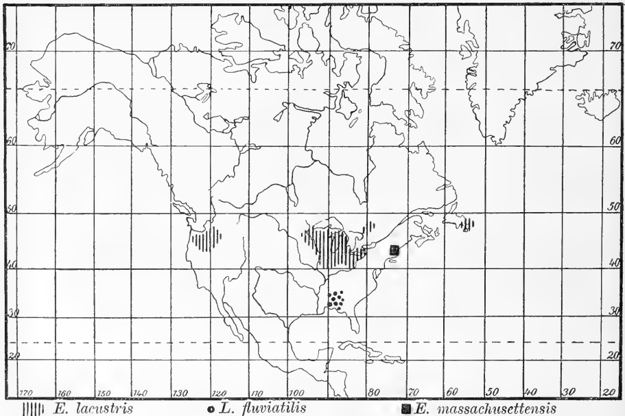
Fig. 04. Verbreitungsgebiet von Epischura lacustris , Epischura massachusettsensis und Lamellipodia fluviatilis .
