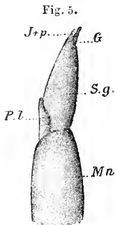
Fig. 5. Velia rivulorum .
