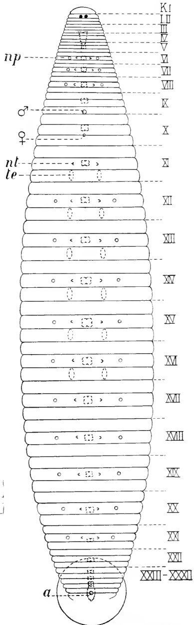
Fig. 1. Clepsine jagerskiöldi .
