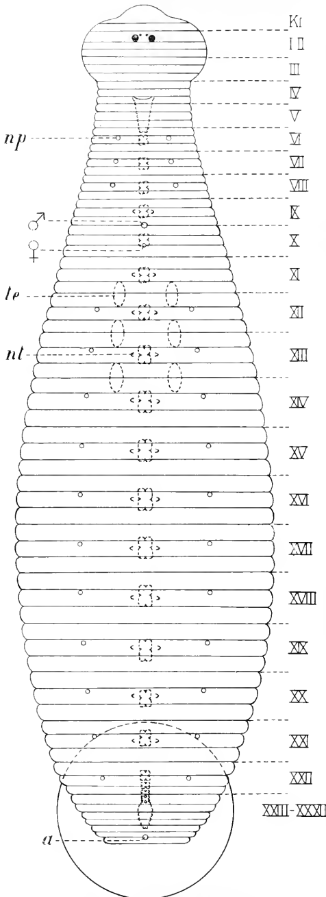
Fig. 3. Clepsine nilotica .
