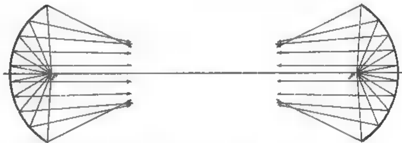
Sphärische Hohlspiegel-Anordnung nach Hansen-Lehmann.
