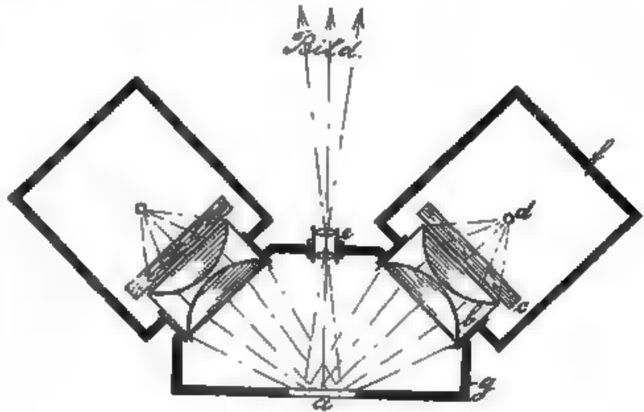
Lichtbild - Apparat (Megaskop) zum Nachweis von Lippenbewegungen.
