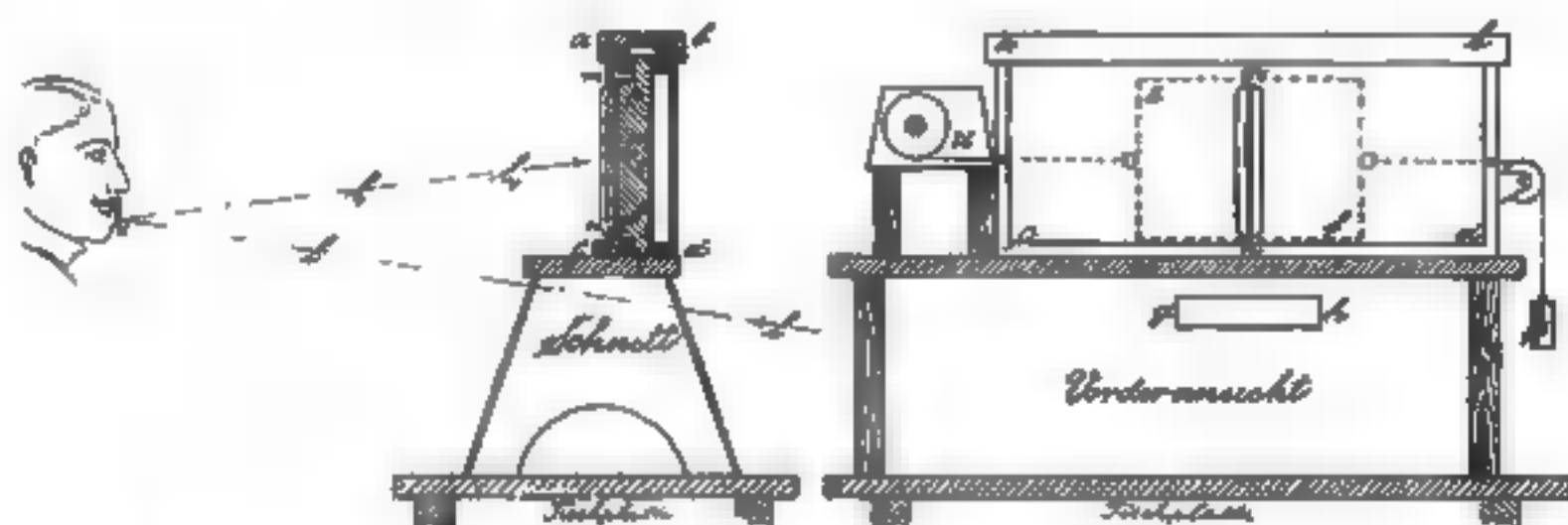
Schnitt durch den Kurven-Apparat. Vorderansicht des Kurven-Apparates
