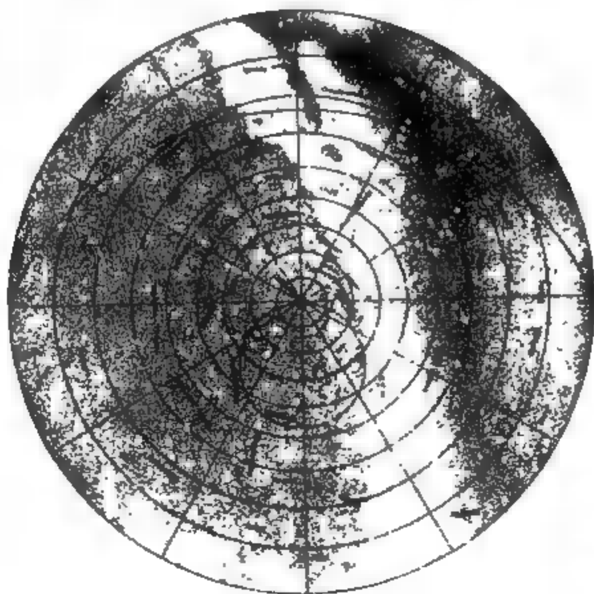
Abb 251 Die Milchstraße auf der südlichen Halbkugel des Himmels
