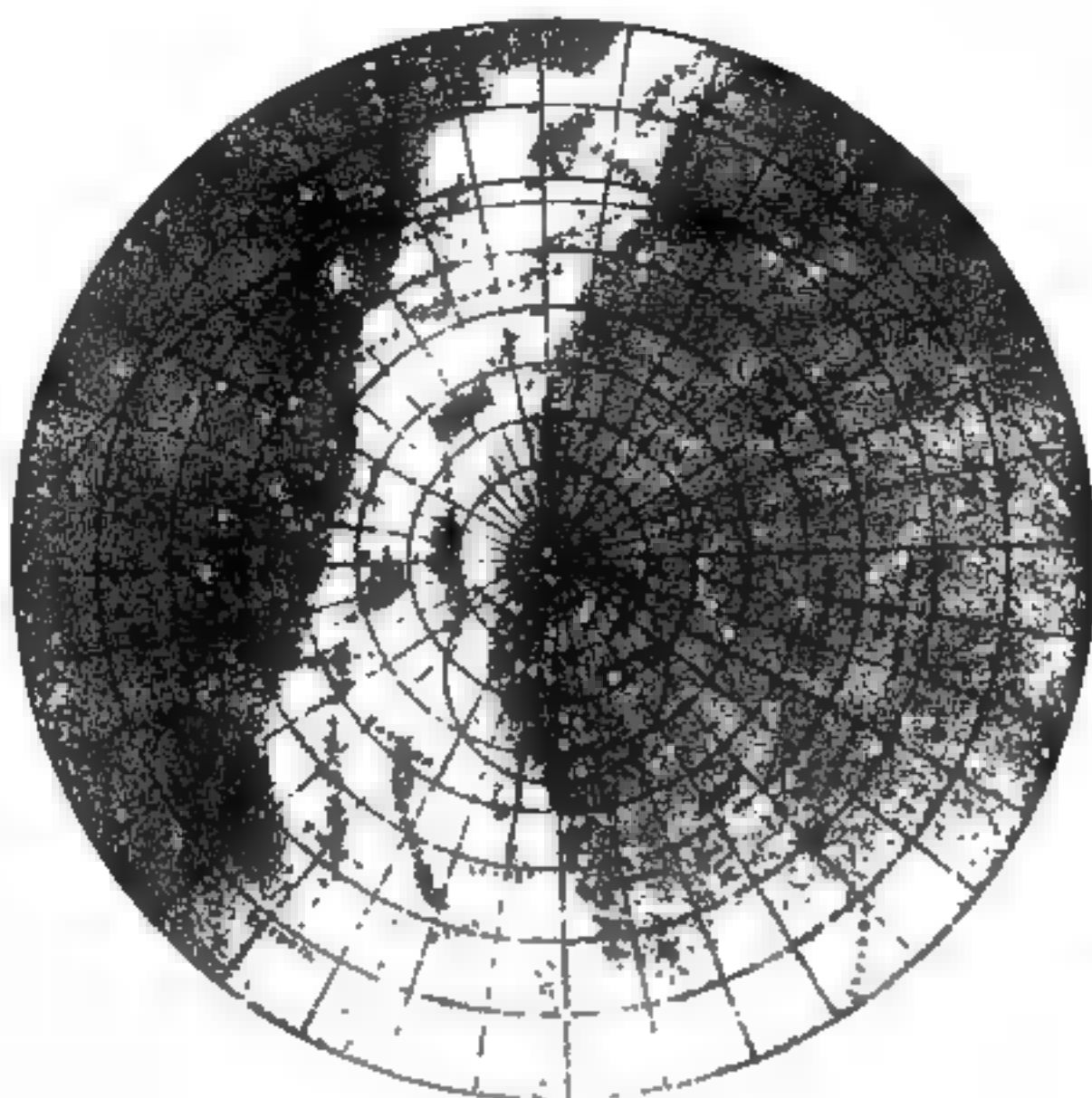
Abb 250 Die Milchstraße auf der nördlichen Halbkugel des Himmels
